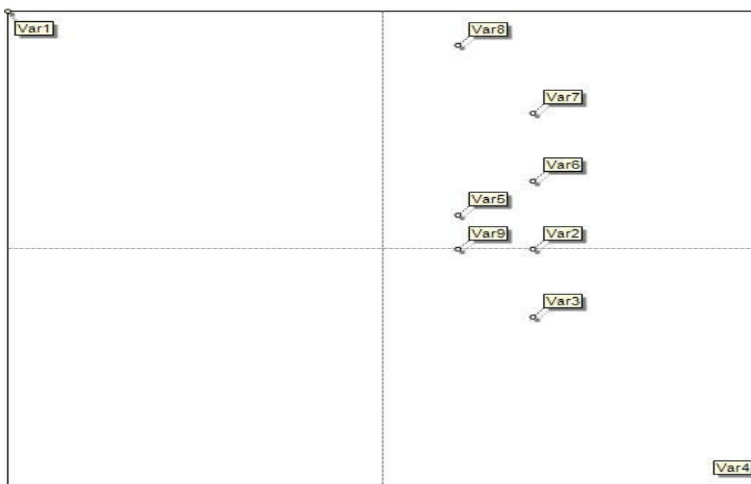
شکل ۲. گراف MICMAC
